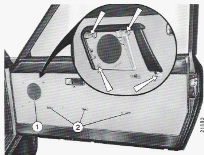
Smontaggio della maniglia per appiglio passeggero.
