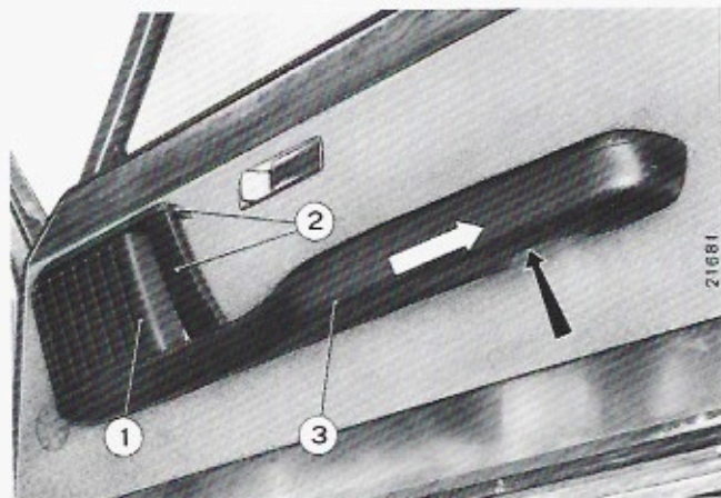
Smontaggio dell'appoggiabraccia dalla porta destra.
